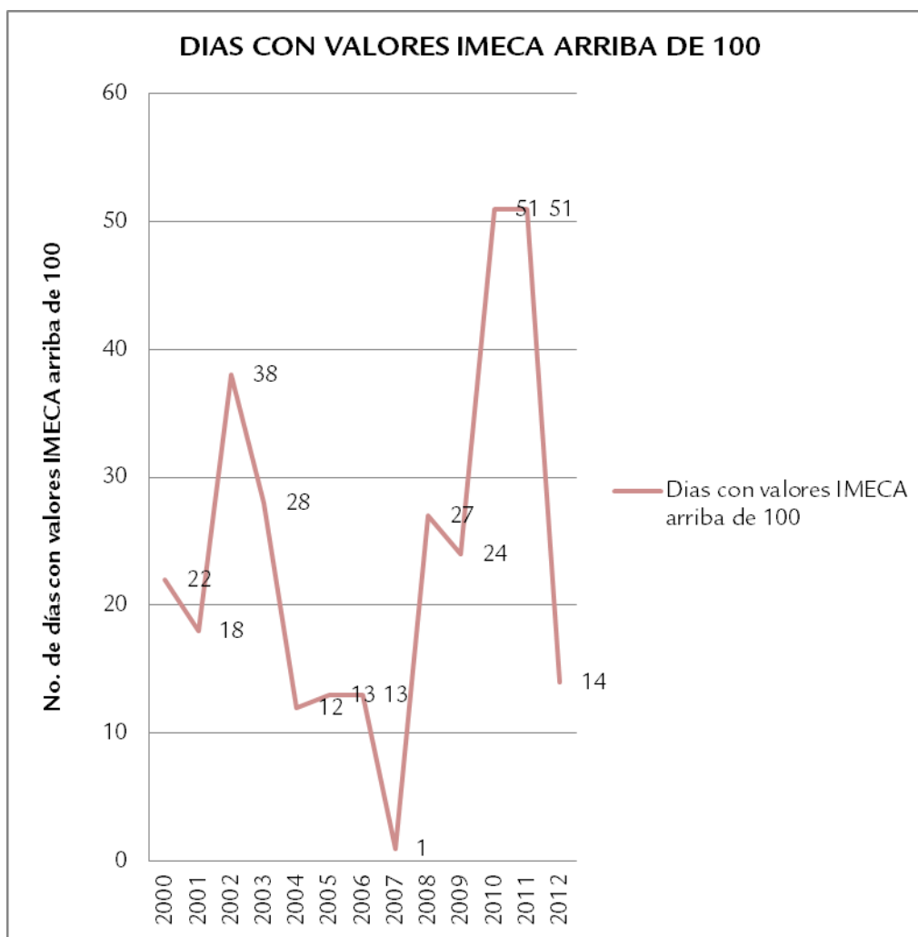
Gráfica 29. Días al año que sobrepasaron los 100 IMECAS en la estación Vallarta.
