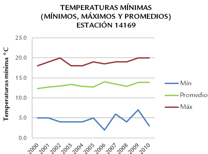
Gráfica 16. Temperaturas mínimas (mínimos, máximos y promedios) por año estación 14169.
