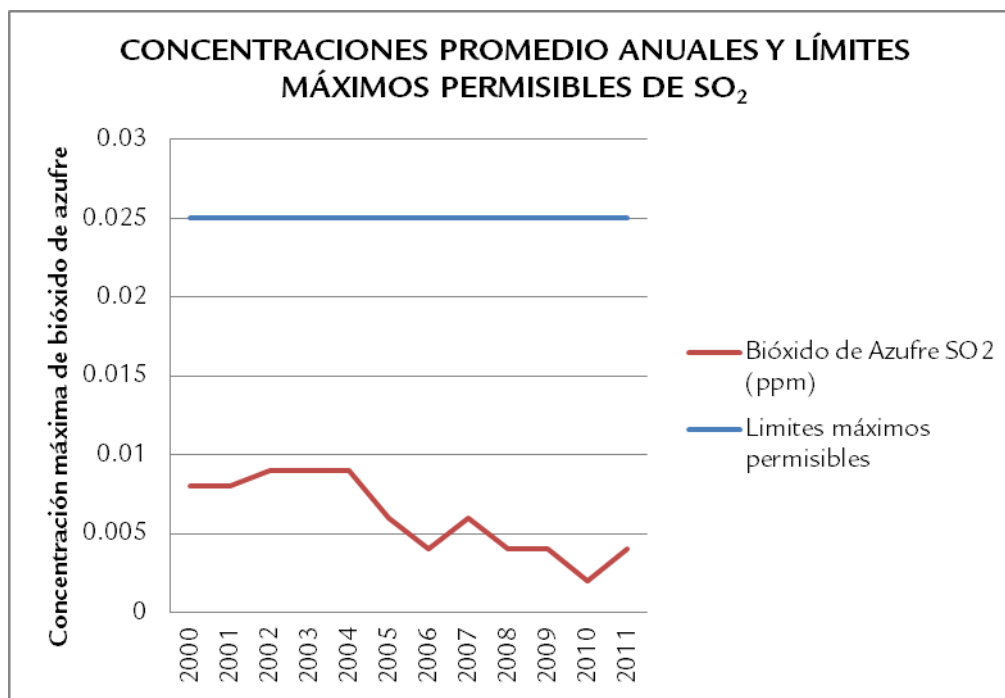
Gráfica 24. Concentraciones promedio anuales de \text{SO}_2 y límites máximos permisibles.
