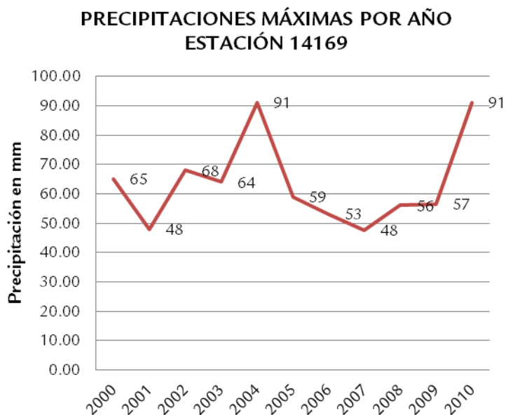
Gráfica 15. Precipitaciones máximas por año estación 14169. Fuente: Elaboración propia con datos SMN.
