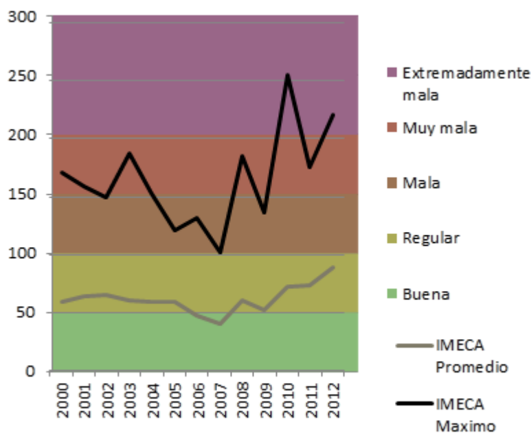
Gráfica 28. IMECAS máximos y promedio anuales.
