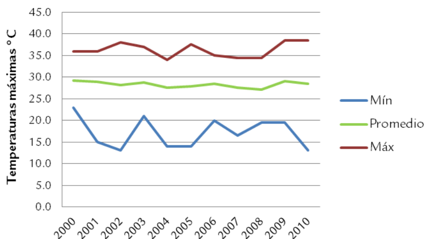
Gráfica 17. Temperaturas máximas (mínimos, máximos y promedios) por año estación 14169.
