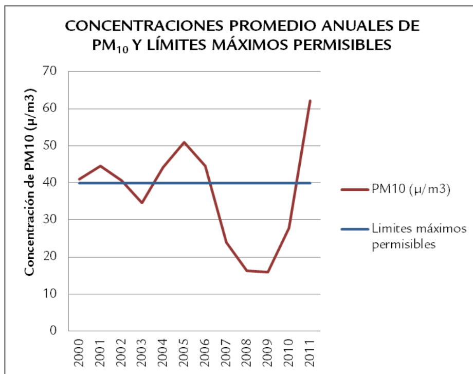
Gráfica 26. Concentraciones promedio anuales de PM 10 y límites máximos permisibles.
