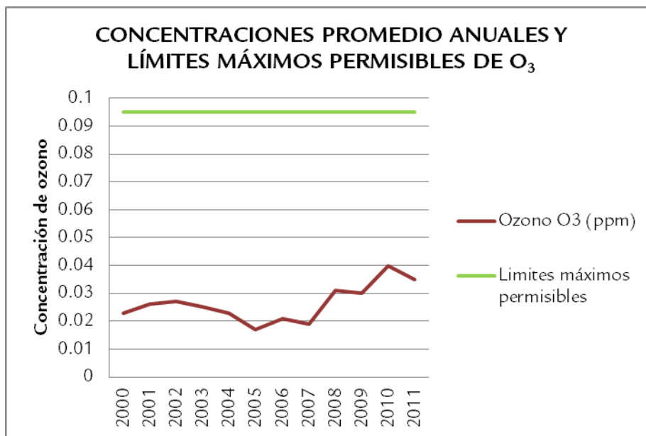
Gráfica 18. Concentraciones promedio anuales y límites máximos permisibles de O 3
