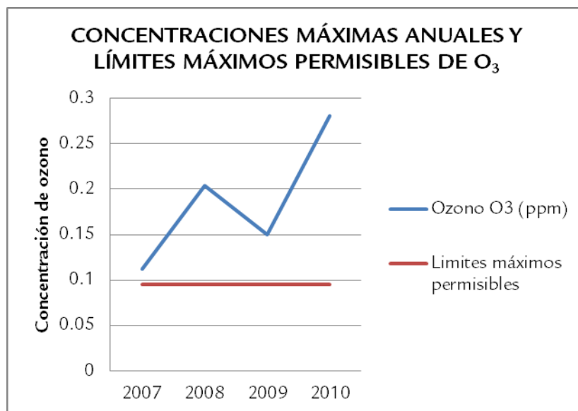
Gráfica 19. Concentraciones máximas registradas por año y límites máximos permisibles de O 3 .
