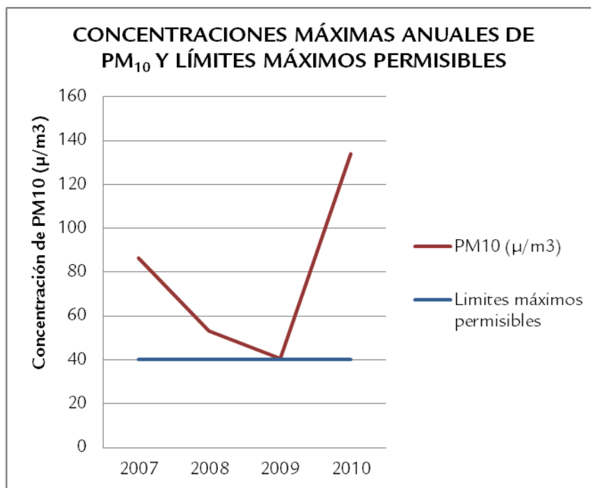
Gráfica 27. Concentraciones máximas anuales de PM_{10} y límites máximos permisibles.
