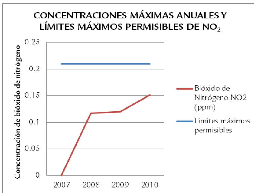
Gráfica 21. Concentraciones máximas anuales de \text{NO}_2 y límites máximos permisibles. Fuente: Elaboración propia con los informes de calidad del aire de SEMADET.
