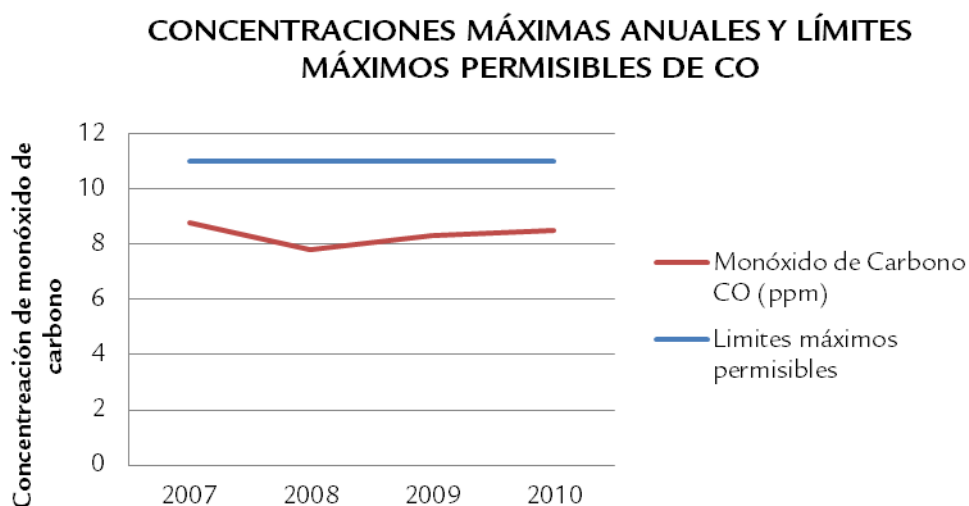
Gráfica 23. Concentraciones máximas anuales de CO y límites máximos permisibles.
