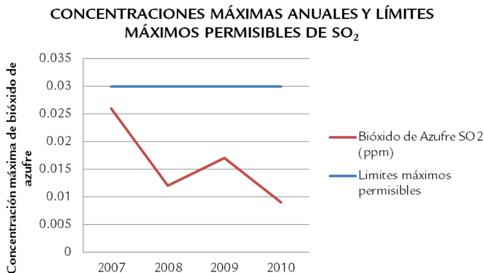
Gráfica 25. Concentraciones máximas anuales de SO 2 y límites máximos permisibles.
