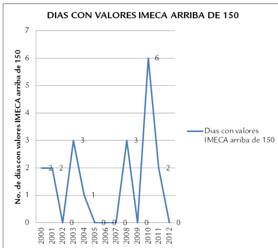
Gráfica 30. Días al año que se rebasaron los 150 IMECAS en la estación Vallarta.
