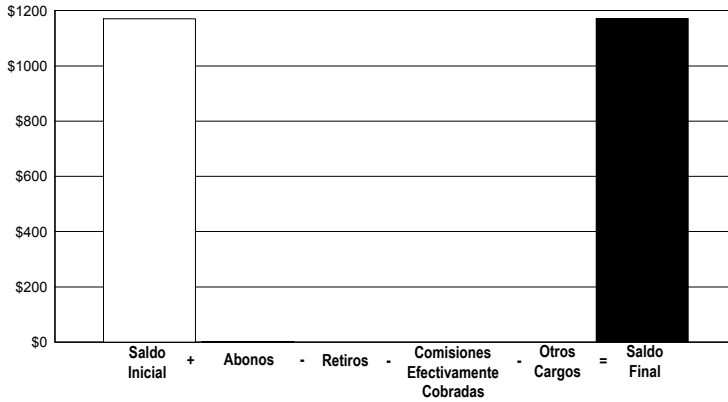
Gráfico Transaccional
