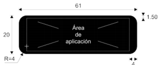
Figura II.2-5. Área de aplicación para la señal SR-37 SENTIDO DE CIRCULACIÓN
