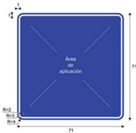
Figura II.5-9. Área de aplicación y dimensiones de los elementos del tablero de las señales turísticas y de servicios
