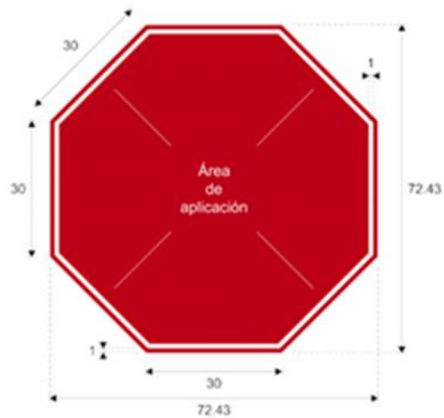
Figura II.2-3. Área de aplicación para la señal SR-6 ALTO
