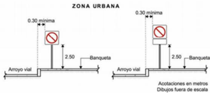
Figura II.2-6. Distancia lateral y altura de las señales restrictivas
