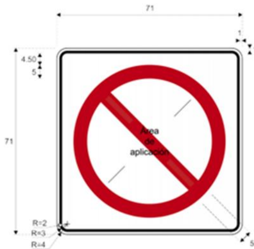
Figura II.2-2. Área de aplicación para las señales restrictivas cuando incluyan una franja diametral
