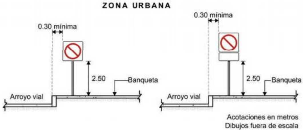
Figura II.2-6. Distancia lateral y altura de las señales restrictivas
