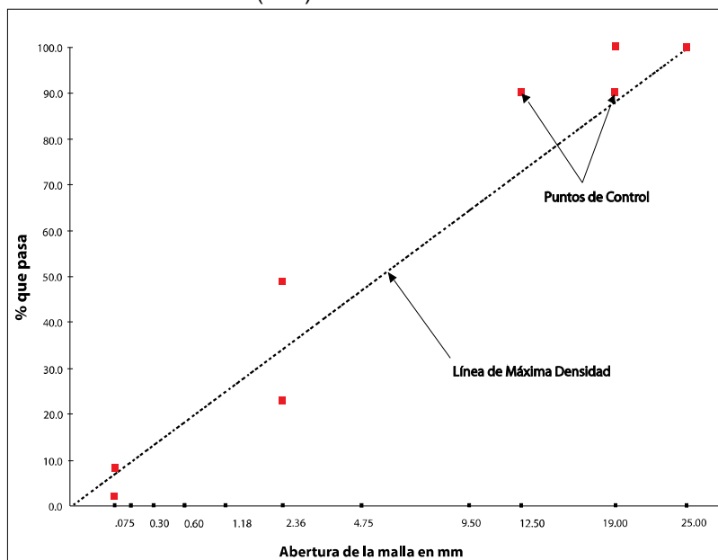
0,45. Gráfica 1.- Granulometría para Mezclas con Tamaño Máximo Nominal 19 mm (3/4”)
